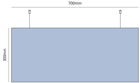
Cat. No. LEF-DS-L-300-700 Unit Size HxW 300mm x 700mm
