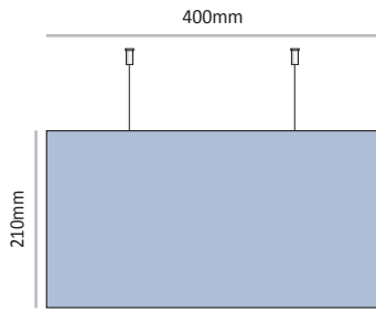
Cat. No. LEF-DS-L-210-400 Unit Size HxW 210mm x 400mm
